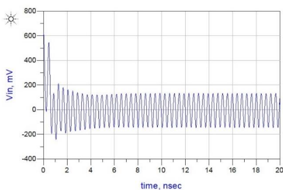
Figure 13. Vin (0 dbm).
